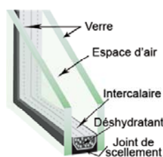
Coupe d'un vitrage isolant
